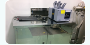
NIR
