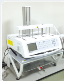
용출시험기
